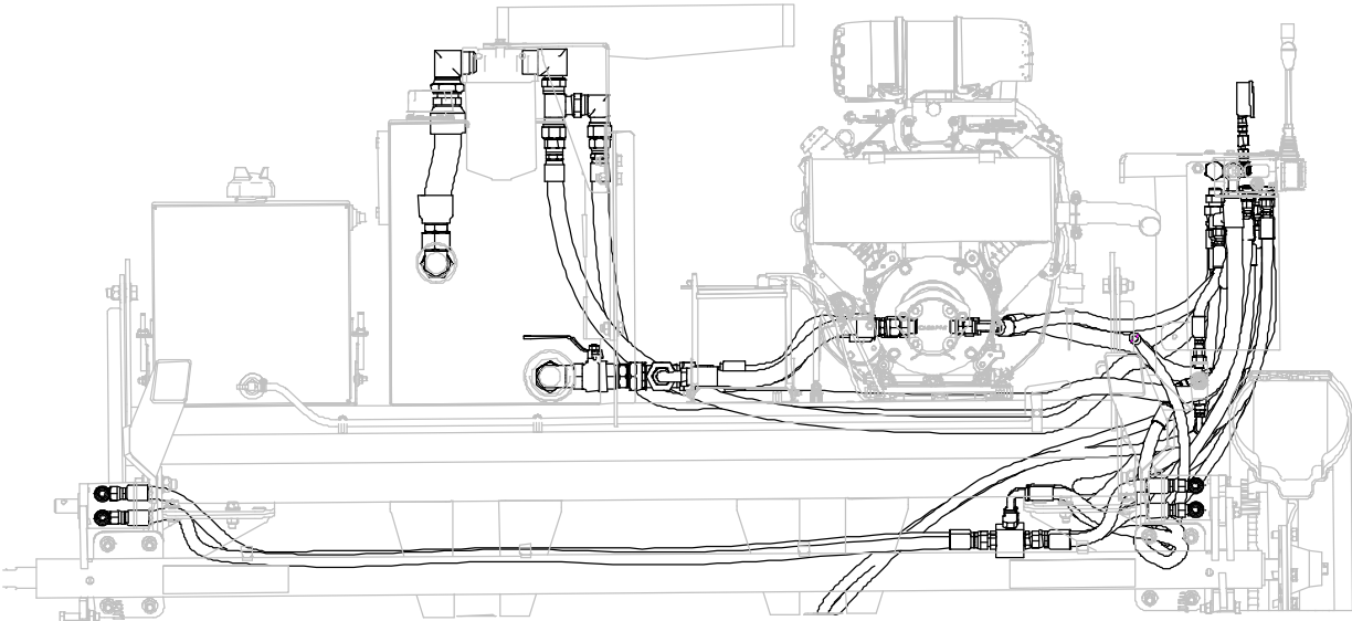
SECTION AJ-AJ
