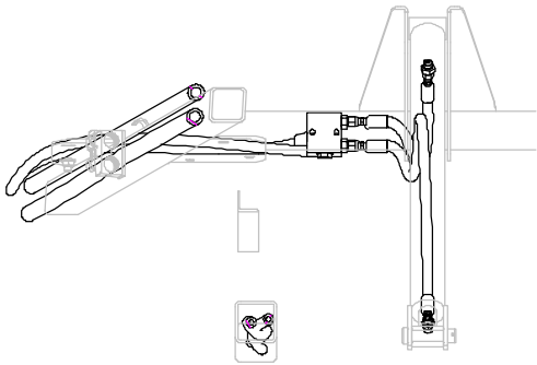
SECTION AK-AK
